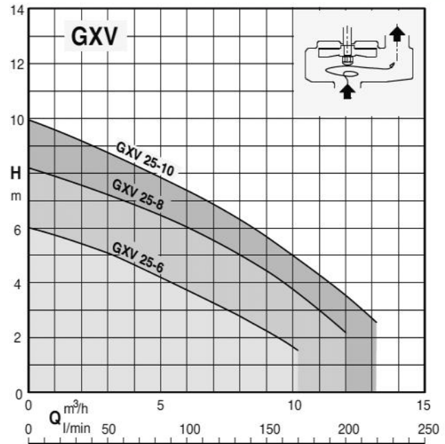
Leistungskennlinien bei 2900 1/min
